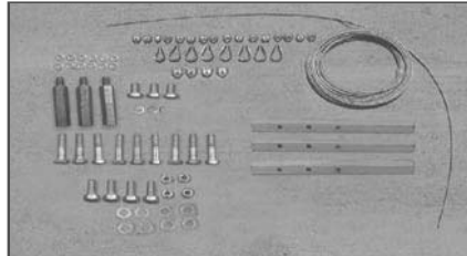
WP Fan Package 16', 24'
