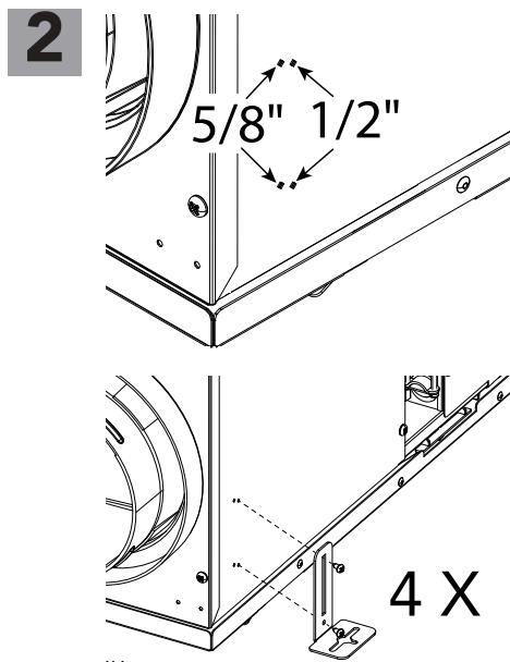
Instalación en la pared
