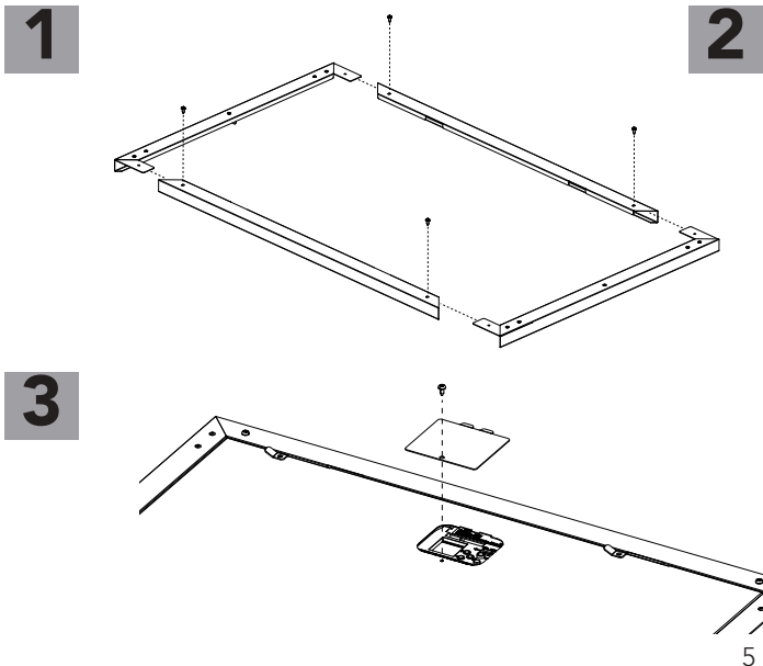
Installation de la bordure
