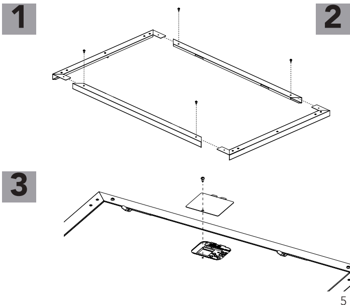
Instalación del borde
