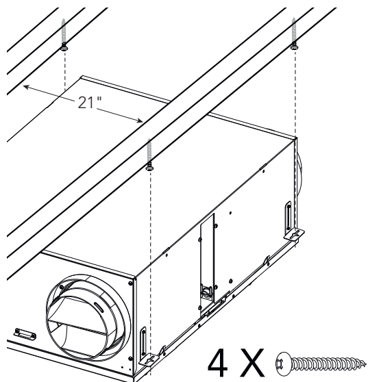
Instalación en techo
